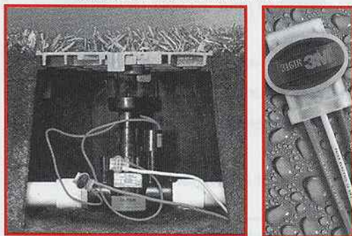
CONNEXION ETANCHE
