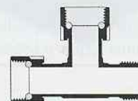
Té union 1" M x 1" F x 1" F
